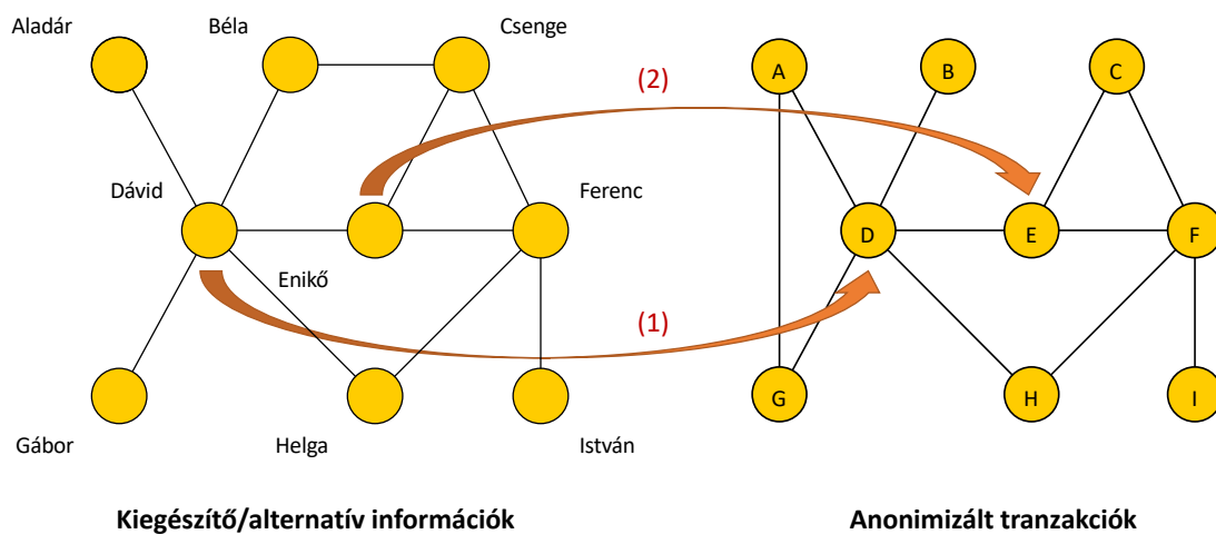
Ábra 2. Egy rosszindulatú harmadik fél próbálkozása a jobb oldalon látható hálózat identitásainak megismerésére. Célja a névtelenül publikált hálózattal együtt megosztott érzékeny információk korlátlan felhasználása az anonimizálás előtti identitások helyreállítása által. Ehhez először globálisan kiugró struktúrájú pontokat keres (1), mint például Dávid. Az ő fokszáma (kapcsolatainak száma) az egész hálózatban egyedi, ami vélhetően teljesül az anonimizált adatban is. A támadó így Dávid kapcsolatba hozza D-vel. Majd ezek környezetében lokálisan kiugrókat (2), mint például Enikő, akinek a fokszáma nem egyedi globálisan, de Dávid környezetében igen.
