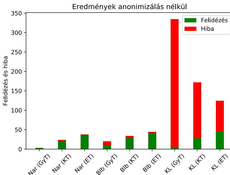
Ábra 11. Anonimizáció nélküli, perturbációval előállított adatokon elért de-anonimizálási eredmények.
