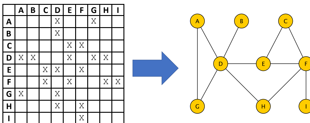
Ábra 1. A tranzakciók táblázata (relációs táblája) értelmezhető egy mátrix szomszédossági mátrixa
