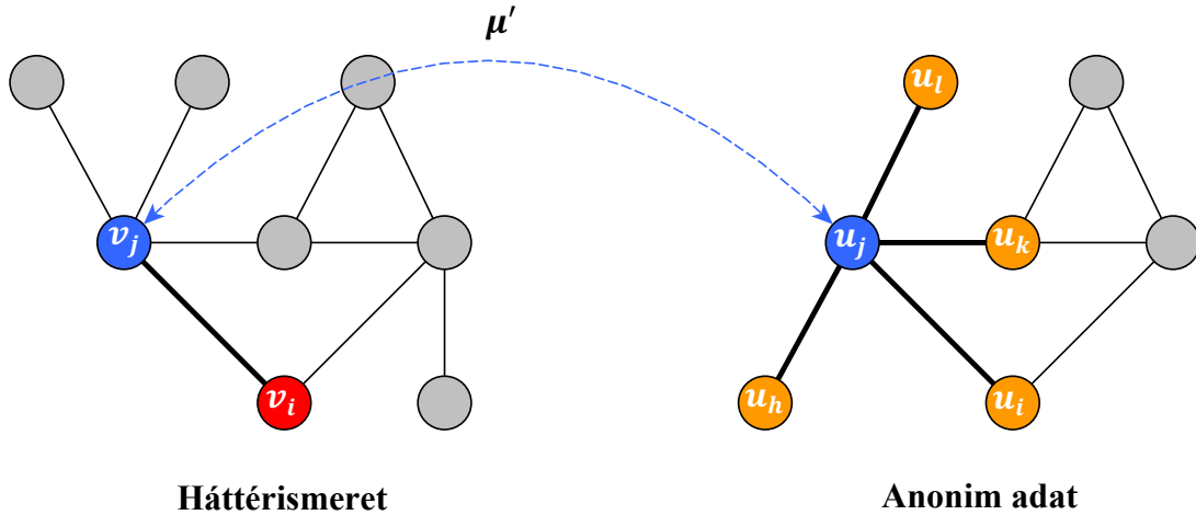
Ábra 9. Alapelv a meglévő hozzárendelések felhasználására az újraazonosítás folyamatában. Ha keressük egy csúchoz a megfelelő hozzárendelést (piros), akkor a vele szomszédos, már hozzárendeléssel bíró csúcsok (bal kék) hozzárendeltjének (jobb kék) a szomszédai között (narancs) keressünk.
