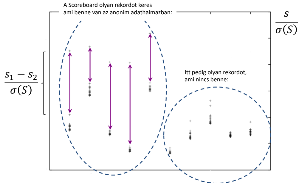
Ábra 6. Magyarázat a kiugróság mérésének jelentőségére a Netflix által publikált adatokon. Az x tengelyen különböző ismert rekordok helyezkednek el, az y tengelyen pedig az ezekhez tartozó hasonlósági mérések eredményei az anonimizált adathalmaz rekordjaihoz képest. Az ábra jól szemlélteti, hogy az anonimizált adatbázisban is szereplő rekordok kiugrósága jelentősen eltér azokétól, amelyek abban nem szerepelnek. (az ábra forrása: [16])
